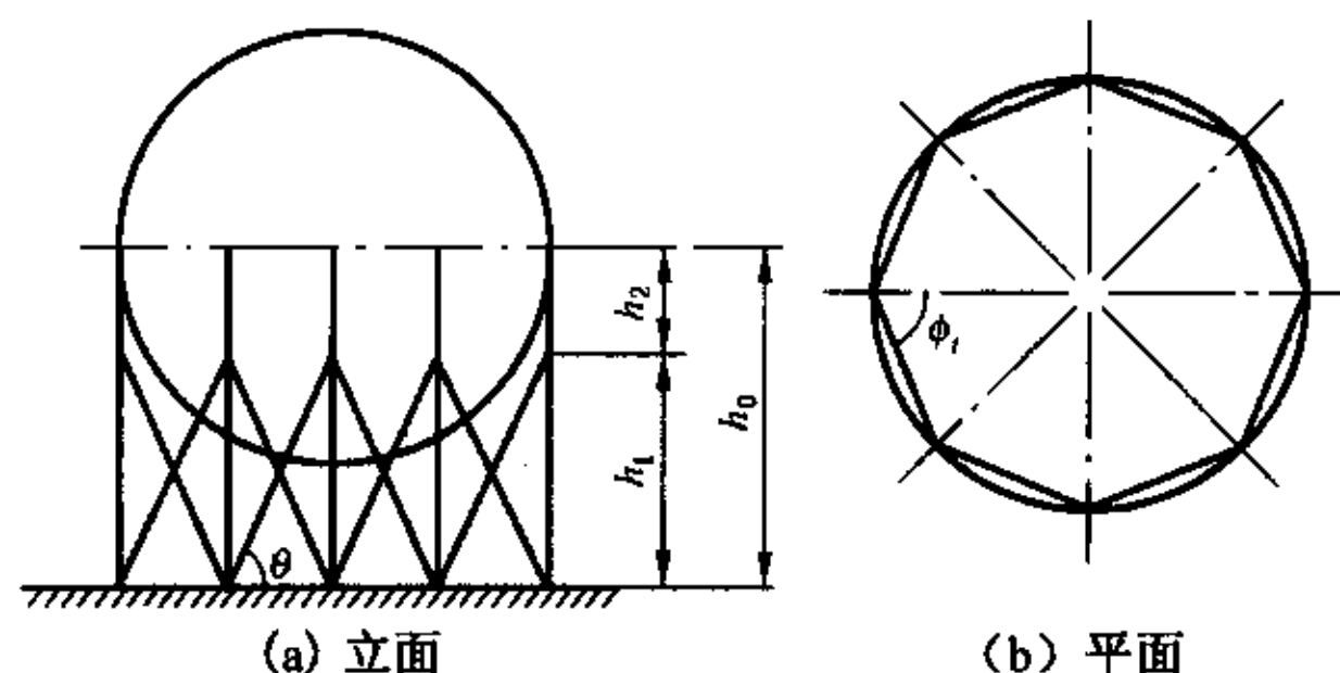
图 7.2.3 球罐简图
