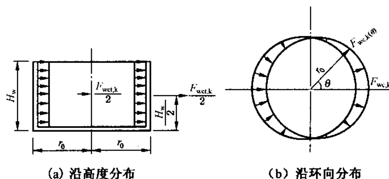
图 6.2.2 圆形水池动水压力
