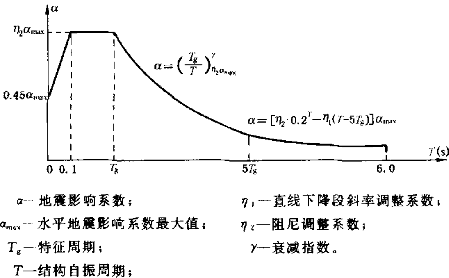
图 5.1.5 地震影响系数曲线
