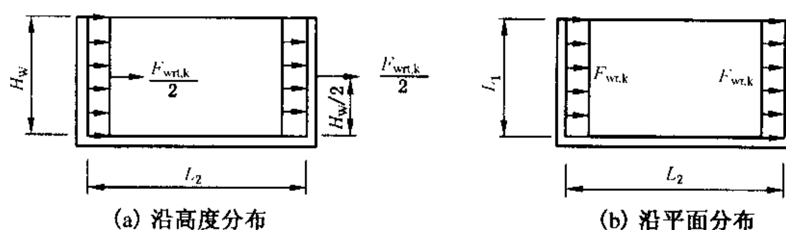
图 6.2.3 矩形水池动水压力
