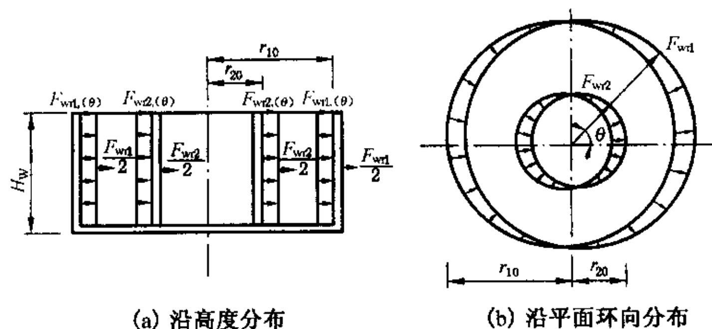
图 7.4.4 环形水槽动水压力
