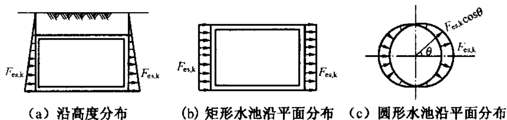
图 6.2.4 动土压力分布图
