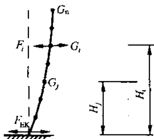
图 5.2.1 水平地震作用计算简图
