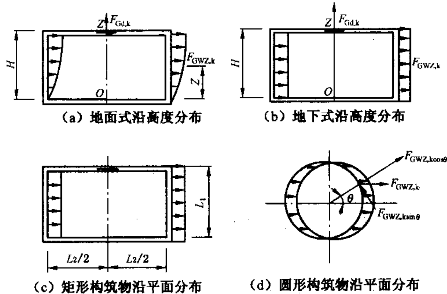
图 6.2.1 自重惯性力分布图
