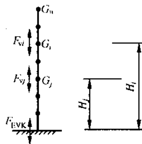
图 5.3.1 结构竖向地震作用计算简图
