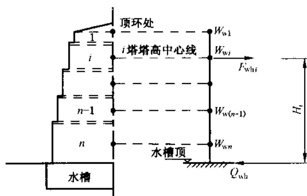
图 7.4.1 湿式罐结构计算简图
