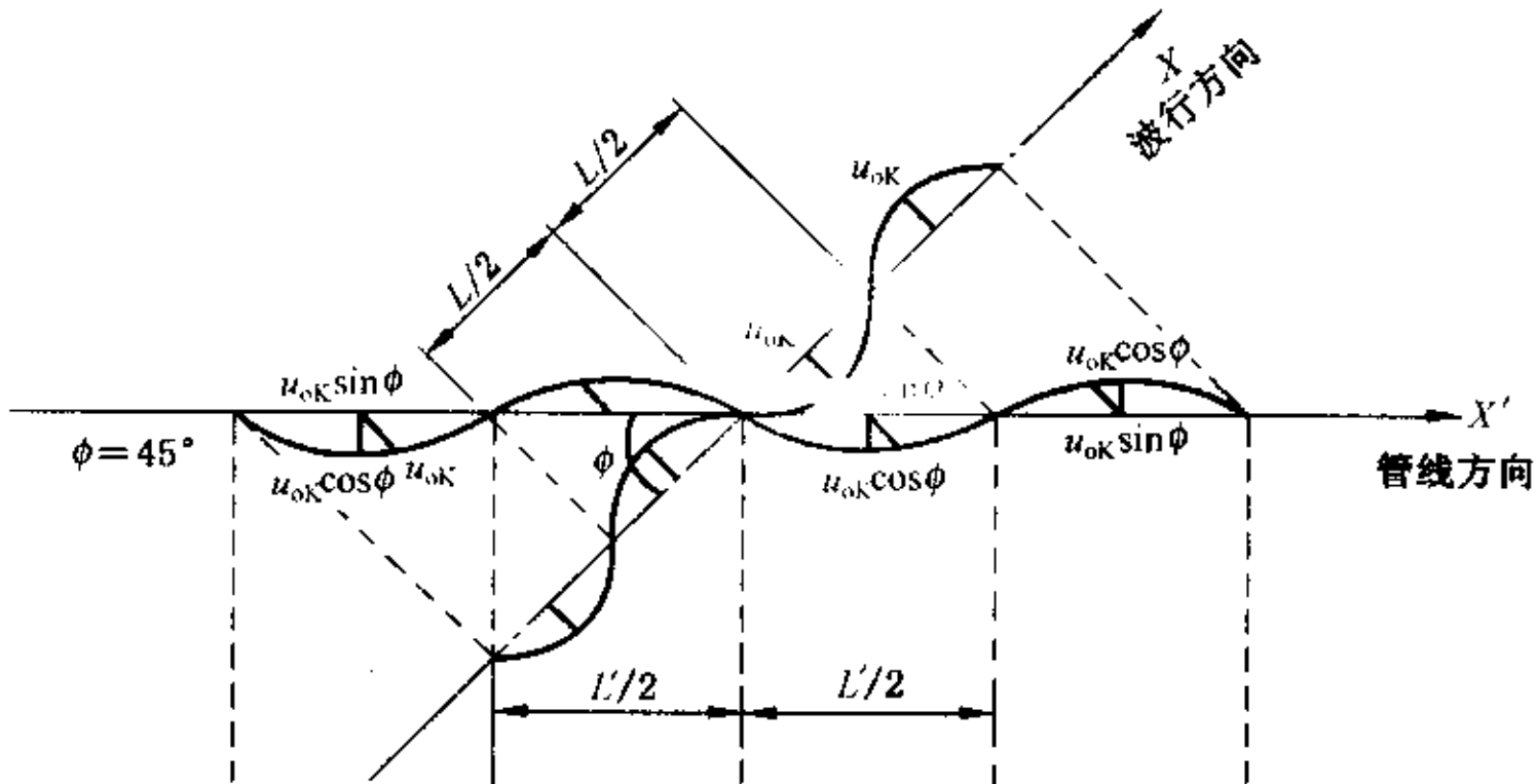
图 C. 1. 1 地下管道计算简图
